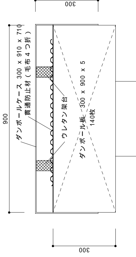
平断面図
